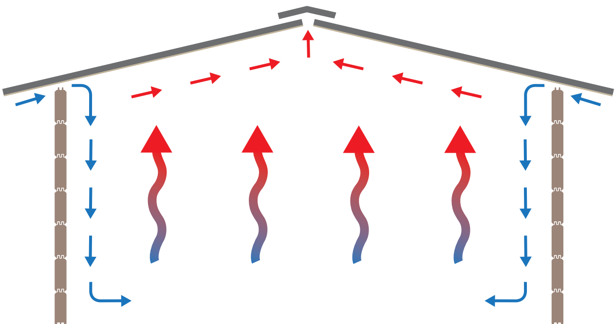
Une ventilation efficace (les flèches montrent que l'air est évacué de la structure.)
