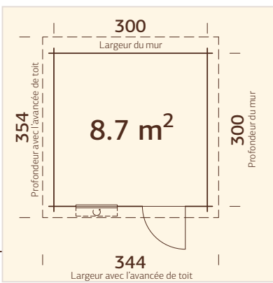
Plan au sol
